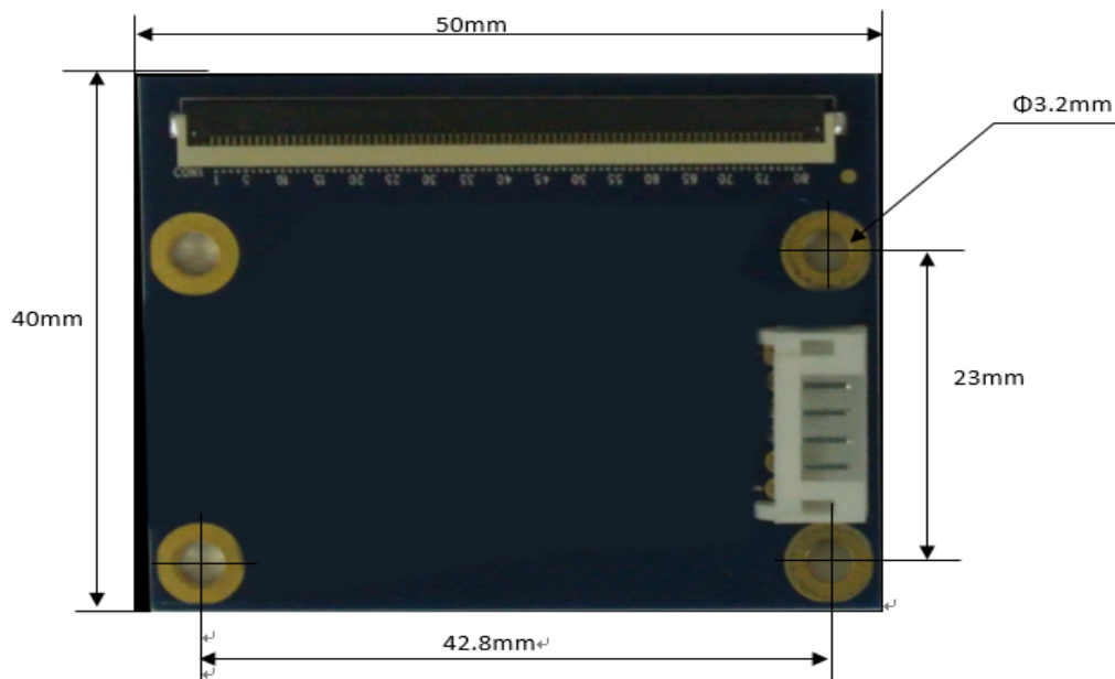
MTX-80 コントローラーサイズ
